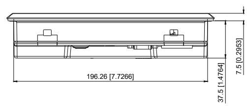
俯视图 (单位: mm, [ ]: inch)
