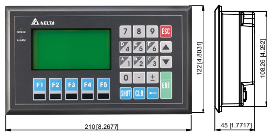
正面图及右侧图 (单位: mm, [ ]: inch)
