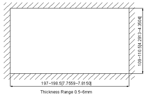
嵌入开孔尺寸 (单位: mm, [ ]: inch)
