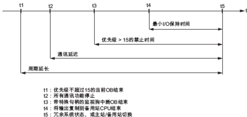
Pic4. 各时间点顺序
