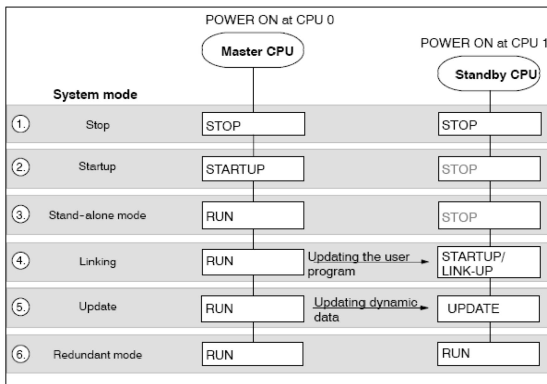
Pic5. 冗余同步过程
