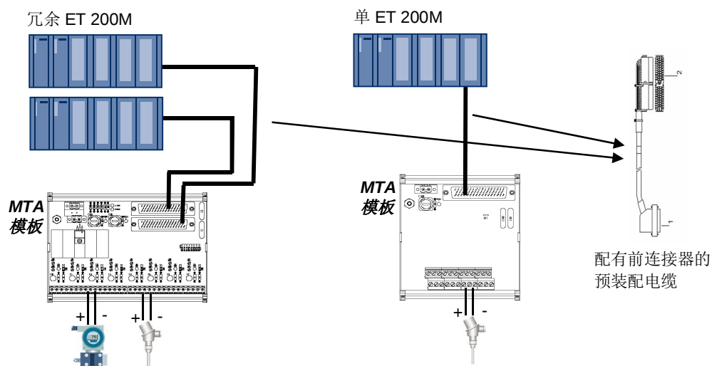
Pic1. MTA应用示意图
