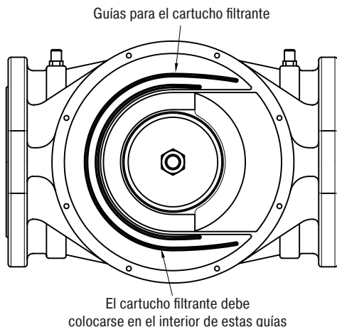
fig. b: Cuerpo DN 65 ÷ DN 100 sin tapa inferior
