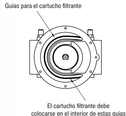
fig. a: Cuerpo DN 15 ÷ DN 50 sin tapa inferior
