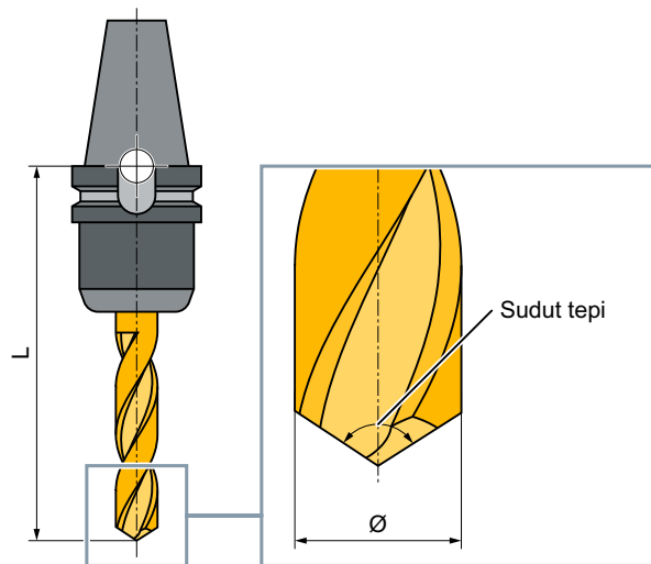
Gambar 12-8 Bor (Tipe 200)
