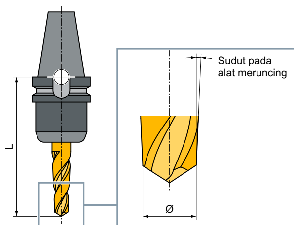
Gambar 12-13 Pahat 3D dengan sebuah contoh pemotong bevel (Tipe 155)
