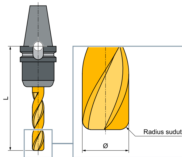
Gambar 12-12 Pahat 3D dengan sebuah contoh frais akhir dengan pembulatan sudut (Tipe 121)
