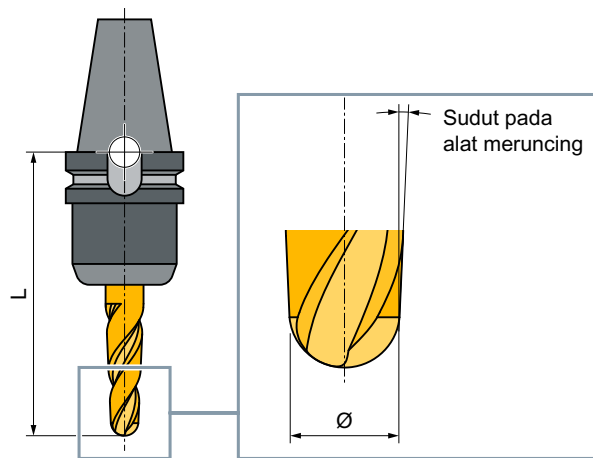
Gambar 12-15 Pahat 3D dengan sebuah contoh pemotong sinking cetakan tekan bertaper (Tipe 157)
