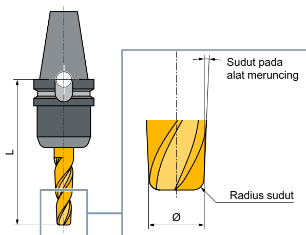
Gambar 12-14 Pahat 3D dengan sebuah contoh pemotong bevel dengan pembulatan sudut (Tipe 156)
