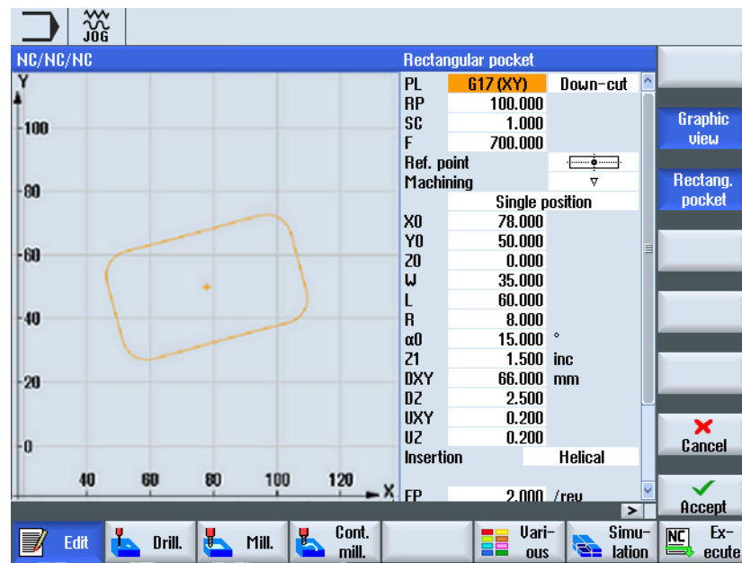
Gambar 9-3 Layar parameter dengan tampilan grafis blok program kode G
