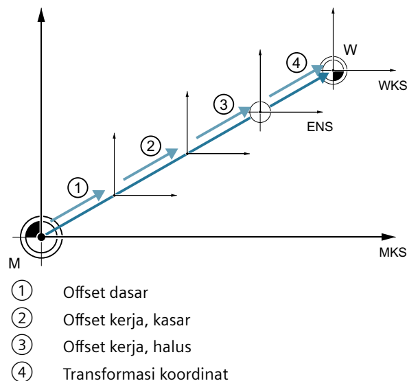
Gambar 5-1 Offset kerja
