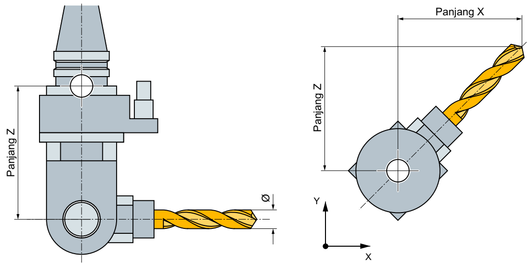
Gambar 12-7 Pemotongan kepala sudut (Tipe 130)
