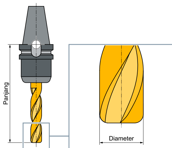
Gambar 12-5 Frais akhir (Tipe 120)
