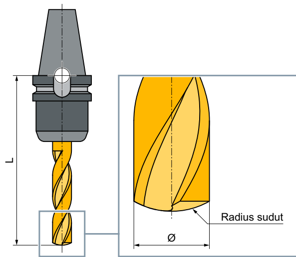
Gambar 12-11 Pahat 3D dengan sebuah contoh pemotong ujung bola (Tipe 111)
