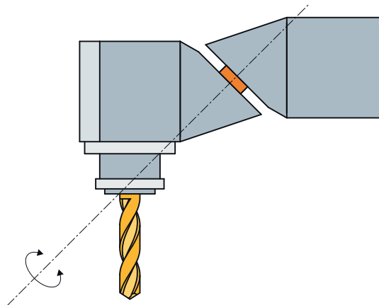
Kombinasi putar 90°/90°
