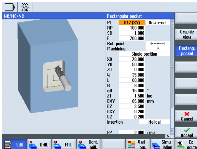
Gambar 9-2 Layar parameter dengan tampilan bantuan
