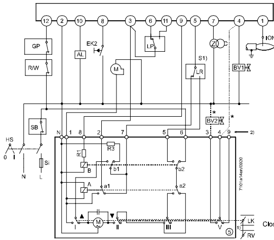
SQL3x.151xx or SQL3x.251xx
