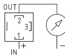
Stromausgang:
