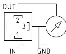
Spannungsausgang:
