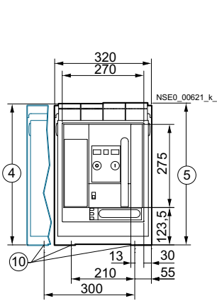
Standardausführung Horizontalanschluss
