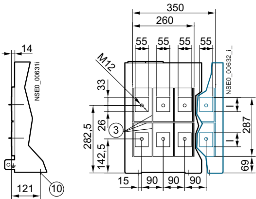
Flanschanschluss
