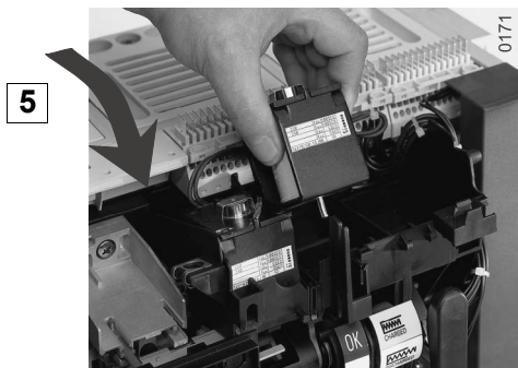
Haltebügel Retaining bracket
