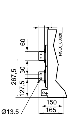
Vertikalanschluss
