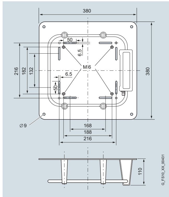
ANT D5 antenna
