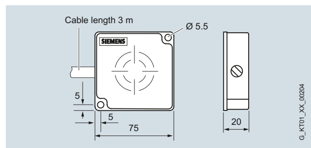
ANT D1 antenna
