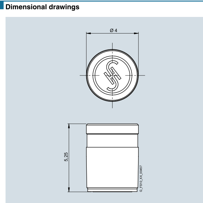
MDS D117 transponder
