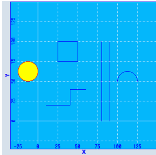
图 9-1 SLEsGraphCustomWidget - 示例
