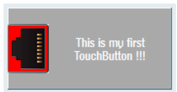
图 9-34 setMargins(0, 0, 0, 0, 0)
