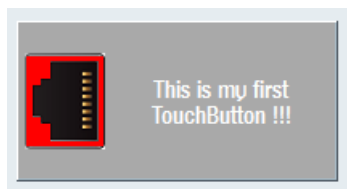
图 9-33 setMargins(-1, -1, -1, -1, -1)
