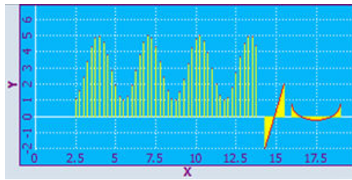
图 9-15 示例 - setIntegralFillMode:关
