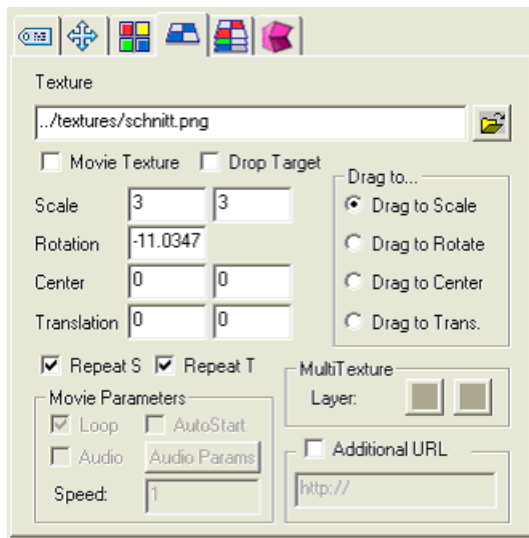
图 C-4 阴影线设置
