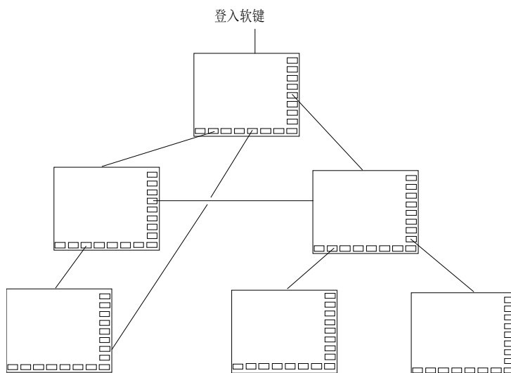
图 5-1 操作树
