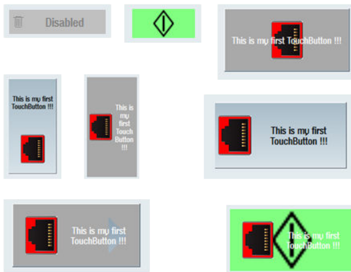
图 9-17 TouchButton 示例
