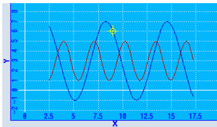
图 9-16 示例 - setCursorOnContour
