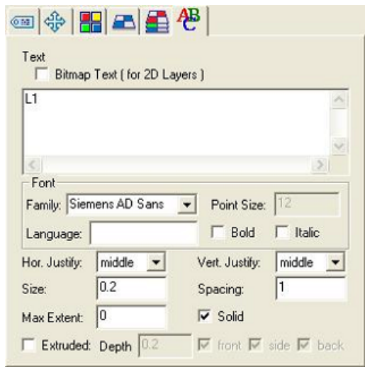
图 C-3 文本设置
