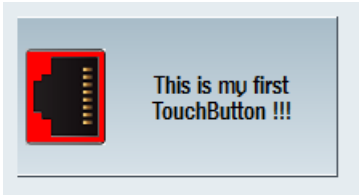
图 9-23 TouchButton 可操作
