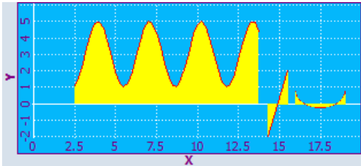
图 9-14 示例 - setIntegralFillMode:开
