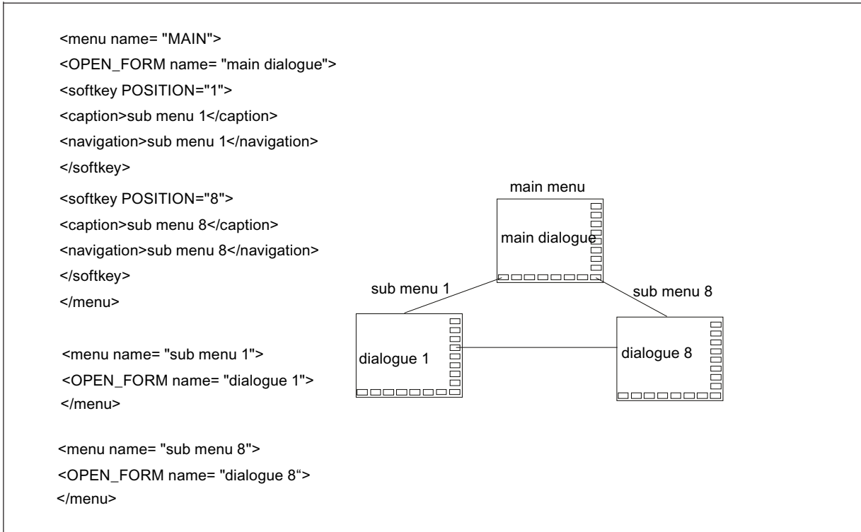
图 3-6 菜单结构
