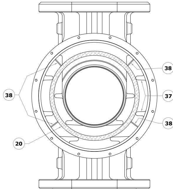
Рис. 12 (вид сверху без крышки). Установите фильтрующий картридж (20), убедившись, что он помещен между специальными направляющими (37), и убедитесь, что ребра (38) хорошо прилегают к корпусу клапана.
