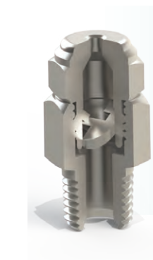
Type SM
