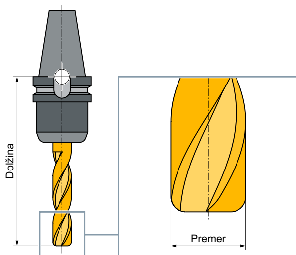
Slika 12-5 Steblasto frezalo (tip 120)
