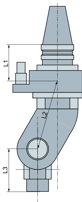
Slika 12-17 Adapter kotne glave
