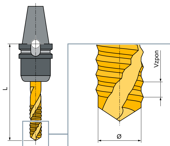
Slika 12-9 Navojni sveder (tip 240)
