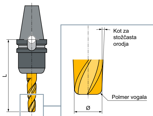
Slika 12-14 3D-orodje na primeru kotnega grezilnega frezala z zaokroženim vogalom (tip 156)
