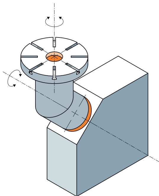
Zasučna miza 90°/45°
