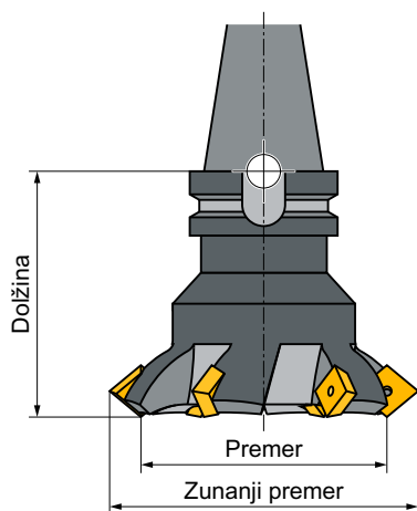
Slika 12-6 Čelno frezalo (tip 140)
