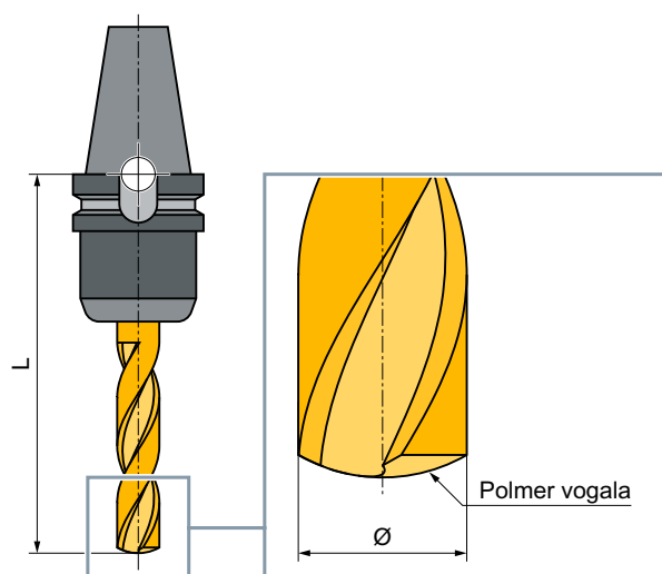
Slika 12-11 3D-tip orodja na primeru krogelnega frezala (tip 111)
