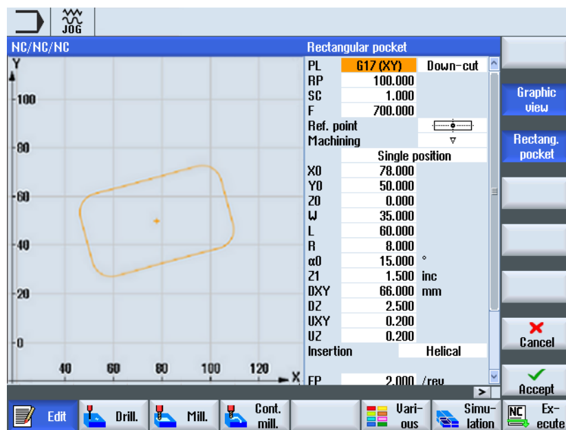
Slika 9-3 Maska parametra z grafičnim prikazom programskega stavka G-kode
