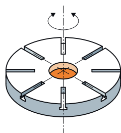
Kombinacija zasuka 90°/90°
