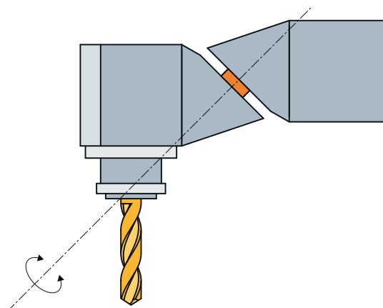
Kombinacija zasuka 90°/90°
