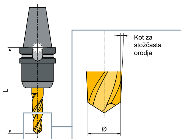
Slika 12-13 3D-tip orodja na primeru kotnega grezilnega frezala (tip 155)
