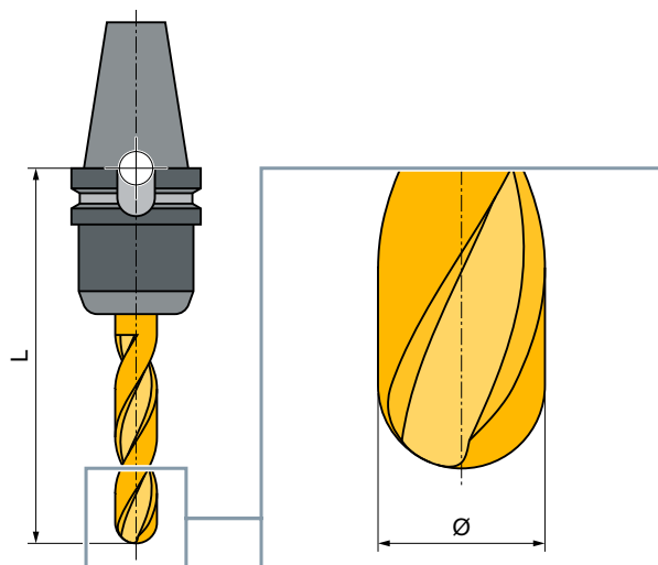
Slika 12-10 3D-orodje na primeru cilindričnega grezilnega frezala (tip 110)
