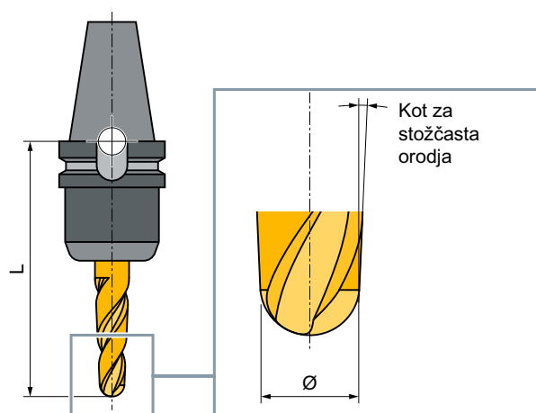
Slika 12-15 3D-orodje na primeru kotnega grezilnega frezala (tip 157)
