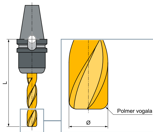
Slika 12-12 3D-orodje na primeru steblastega frezala z zaokroženim vogalom (tip 121)
