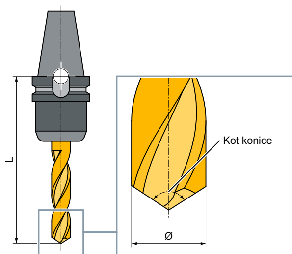
Slika 12-8 Sveder (tip 200)
