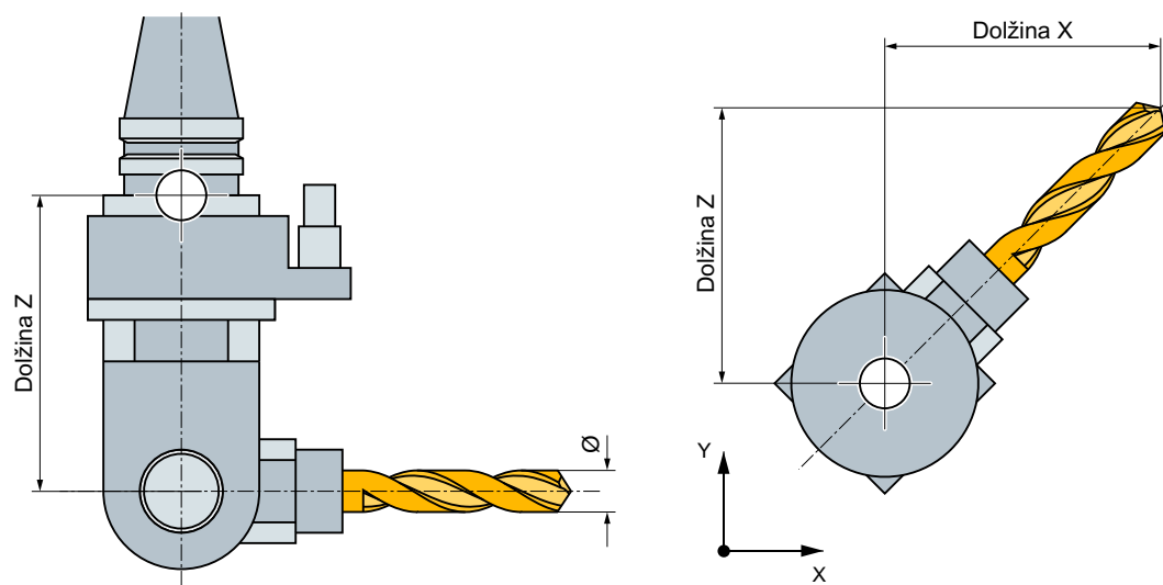
Slika 12-7 Frezalo s kotno glavom (tip 130)
