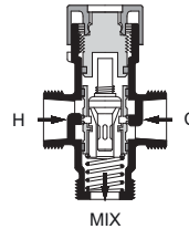
Mischventil
