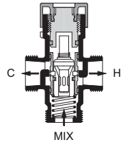
Verteilerventil TM50-1/2E only
