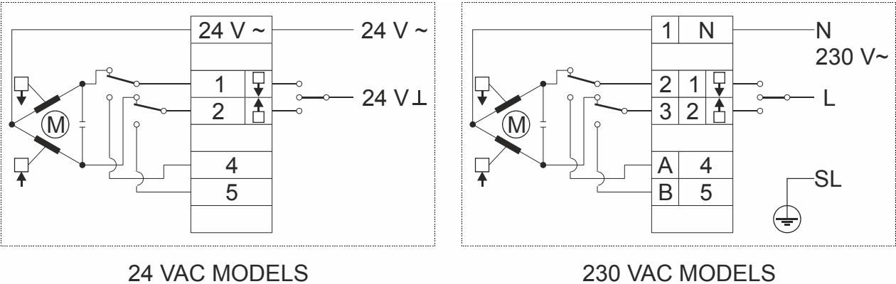
Fig. 3. Wiring
