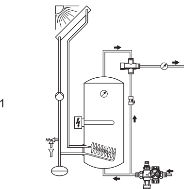
Centrální regulace teploty v solárně vytápěných systémech s dvojím zdrojem energie
