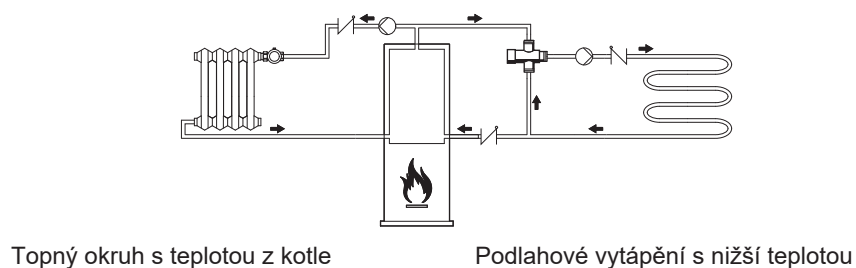
Obr. 1 Příklad standardní instalace směšovacího ventilu
