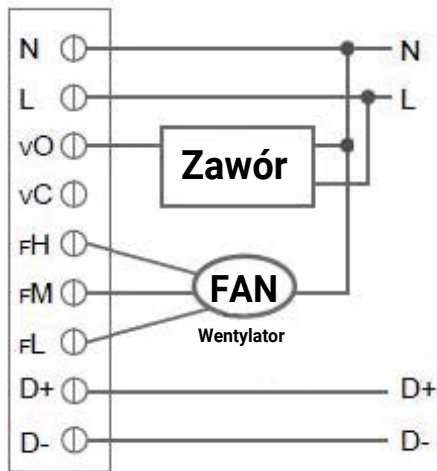
Rys. 2. Napędy SPST
