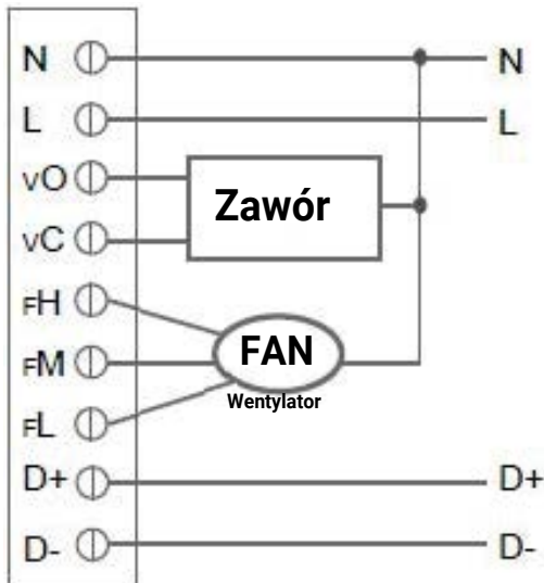
Rys. 3. Napędy SPDT
