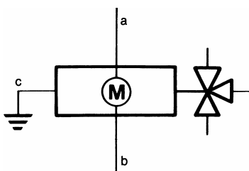
Obr. 3. Diagram připojení ventilu V4044C
