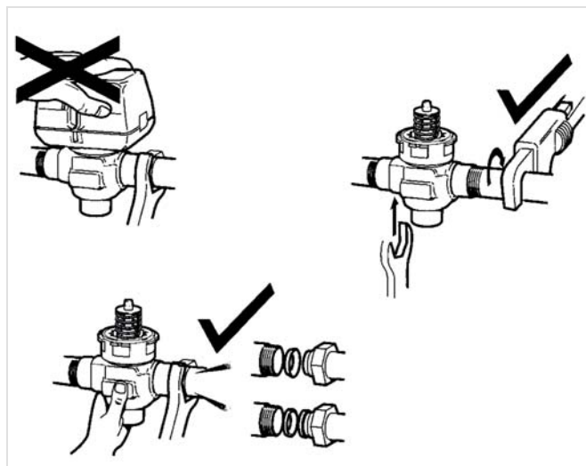
Fig. 5 Raccordement
