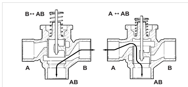
Fig. 2 Débit de fluide à travers une vanne VC à 3 voies
