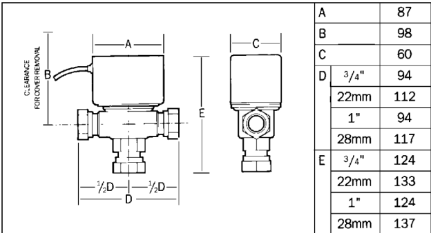
Fig. 1. Dimensions (mm).
