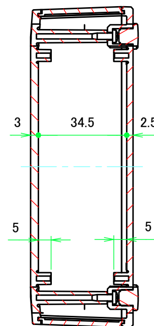
A-A ( 1 : 1.5 )
