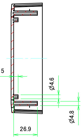
C-C ( 1 : 2 )
