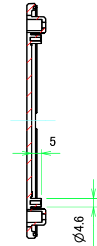
E-E ( 1 : 2 )
