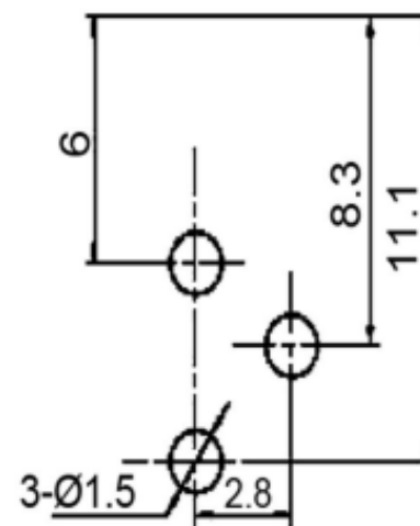
P.C.B LAYOUT
