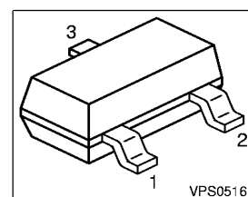
PG-SOT-23
