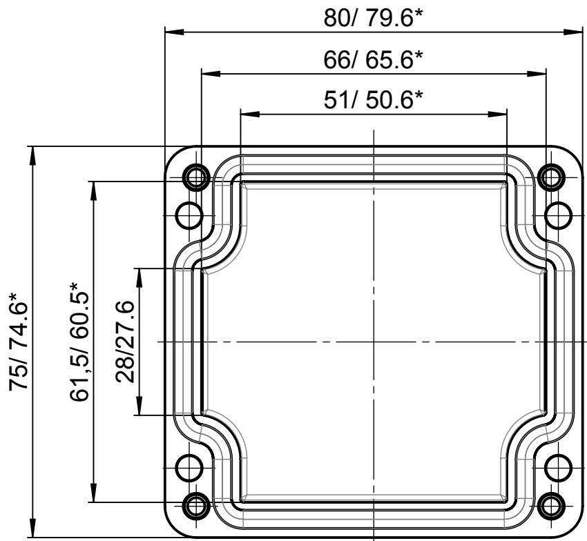
Deckel / lid
