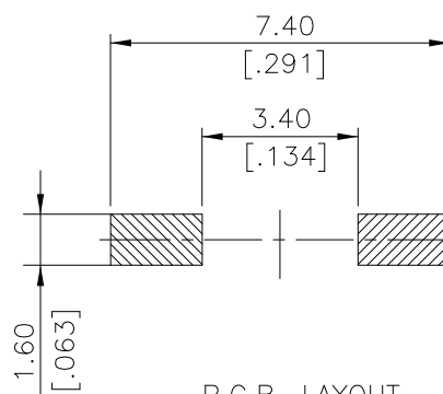
P.C.B. LAYOUT
