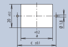
Frontplattenausschnitt · Front Panel Cut-Out
