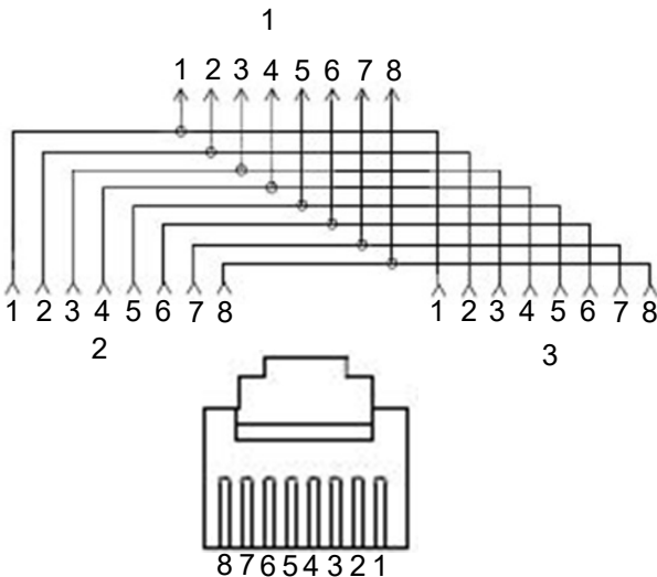
Schaltplan / Wiring diagram
