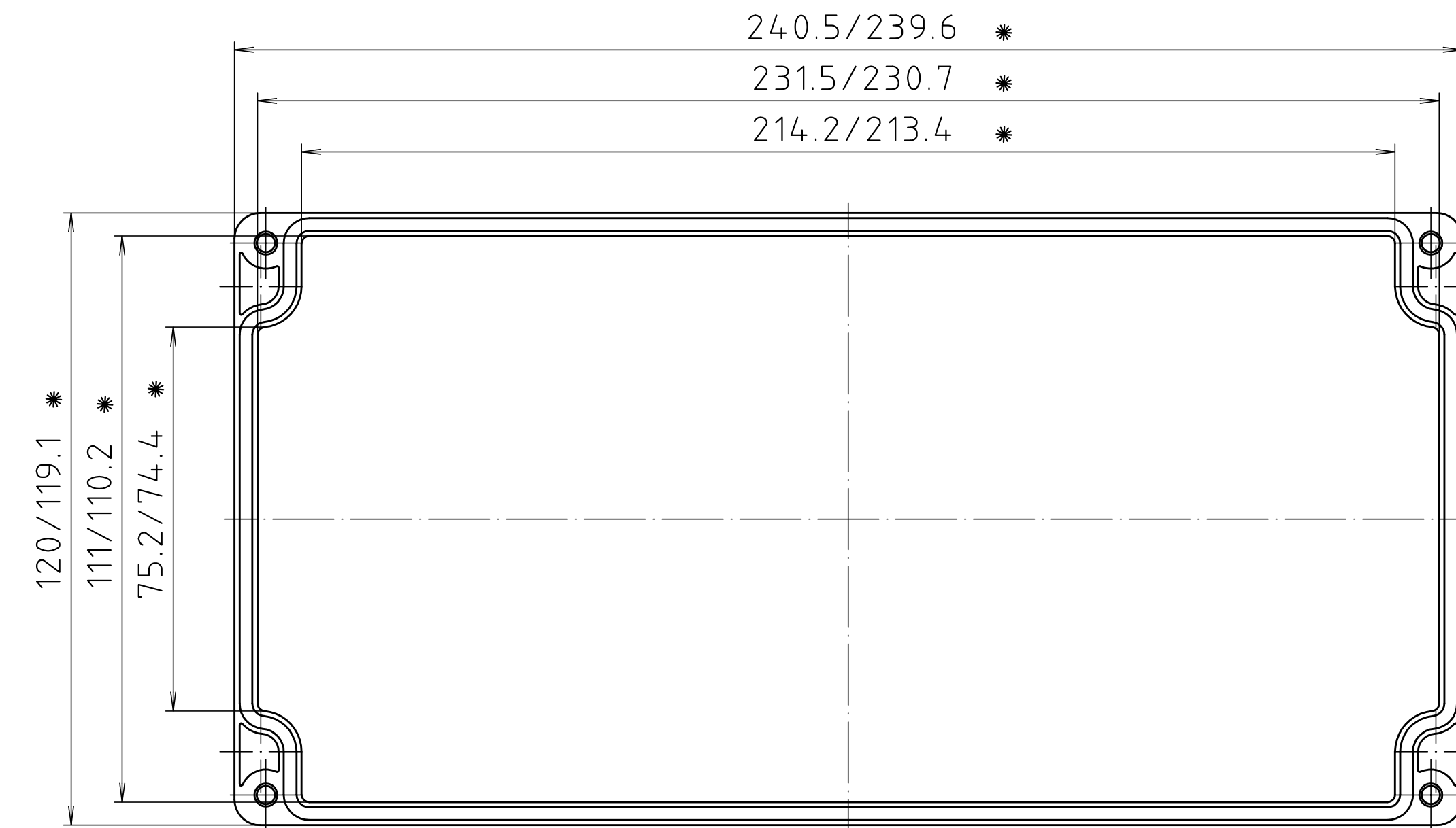
Deckel / lid
