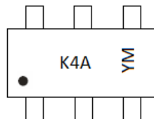
SOT363
