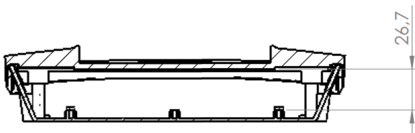
Sección / Section U-U
