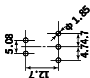
取付穴参考寸法 Mounting Hole
