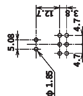
取付穴参考寸法 Mounting Hole
