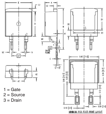
TO-263HV Outline
