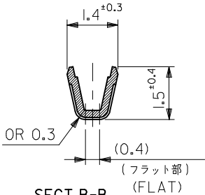
SECT.B-B
