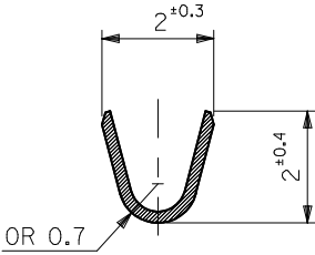
SECT.A-A
