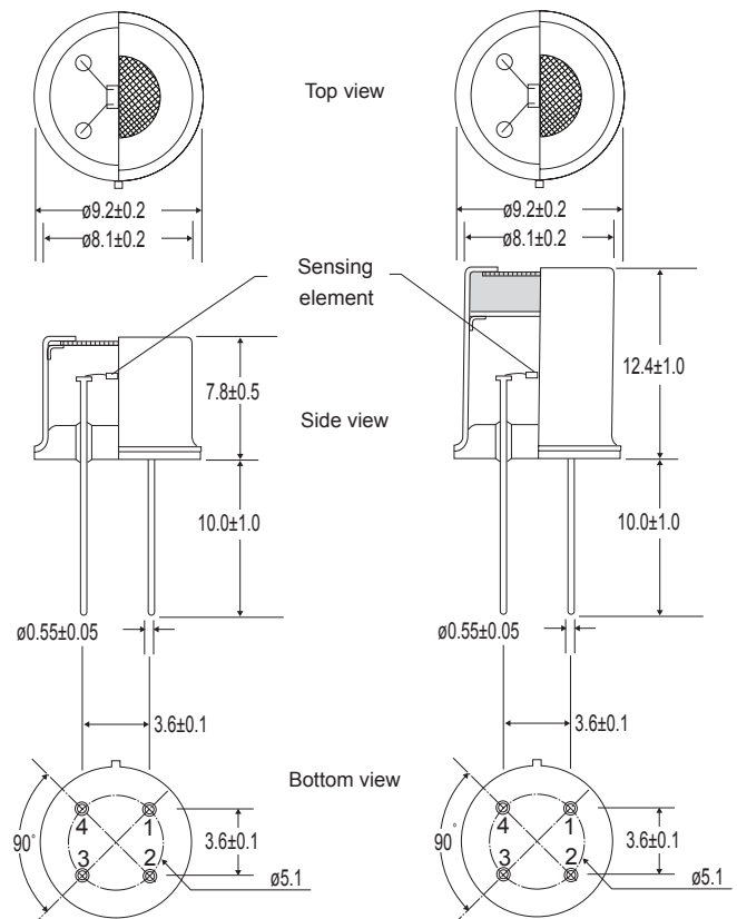
TGS2611-C00
