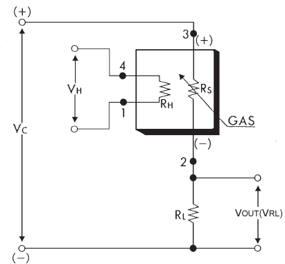
TGS2611-C00
