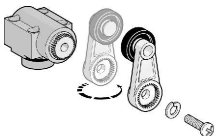
Możliwość obrotu dźwigni z rolką o 180° w łącznikach PAP1, PDP1, PAM1, PDM1, PEM
