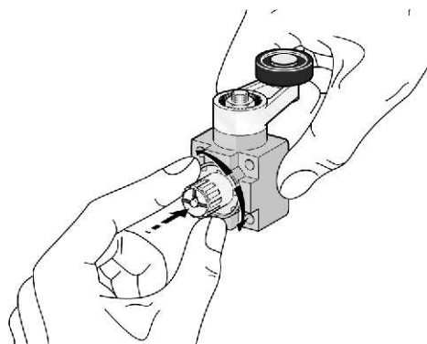
Wybór sposobu działania dźwigni w łącznikach PBM1
