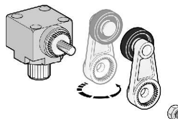
Możliwość obrotu dźwigni z rolką o 180° w łącznikach PBM1
