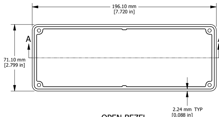
OPEN BEZEL
