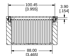
SECTION D-D
