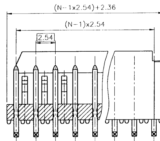
SECTION D-D
