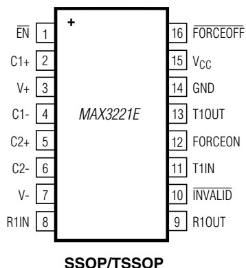
SSOP/TSSOP
