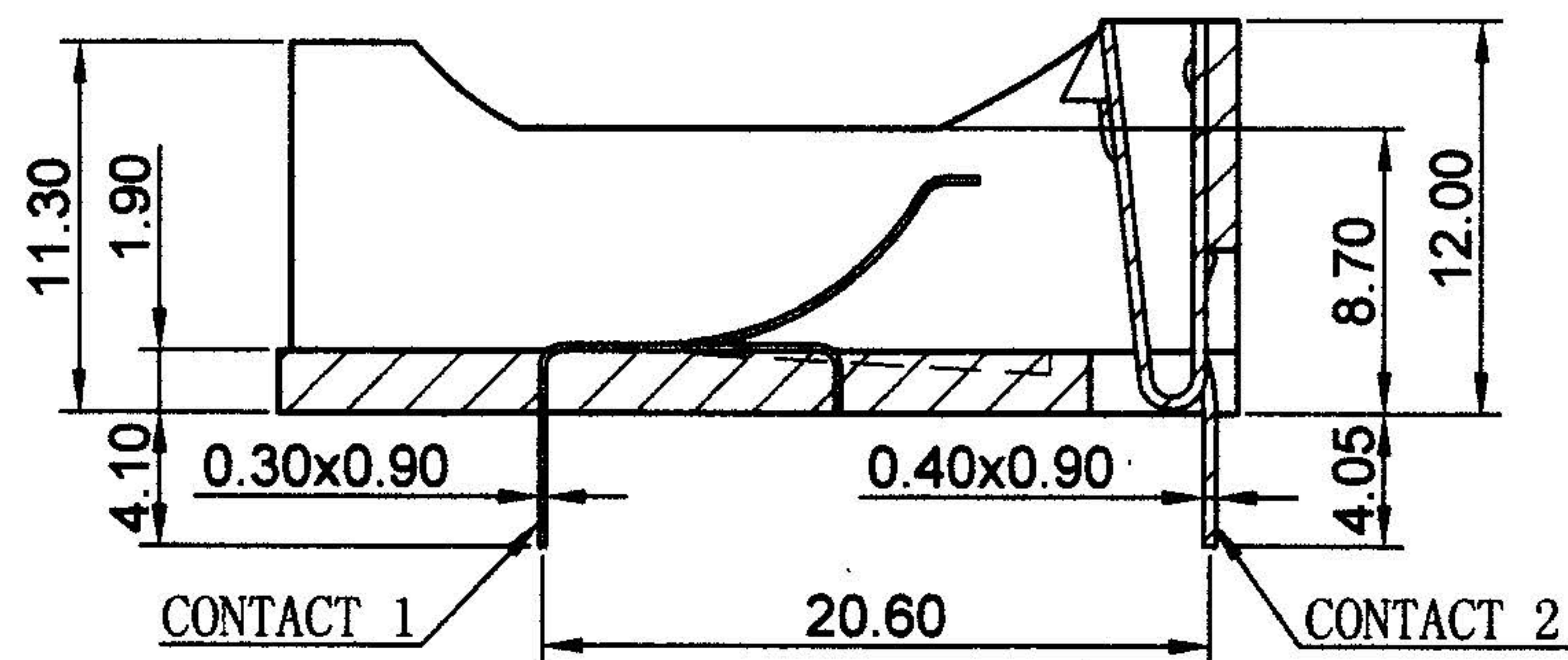
SECTION A-A
