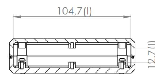
Sección/Section Q-Q
