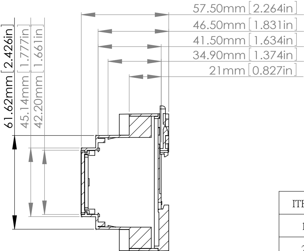
SECTION B-B SCALE 2 : 3
