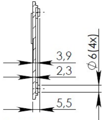
PRZEKRÓJ B-B
