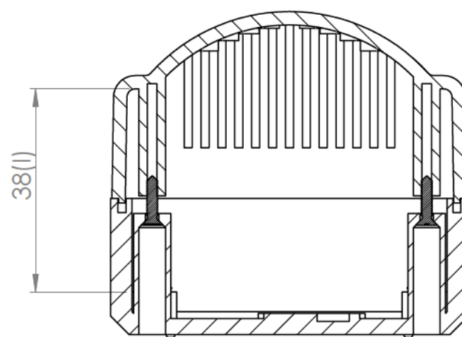
Sección/Section P-P
