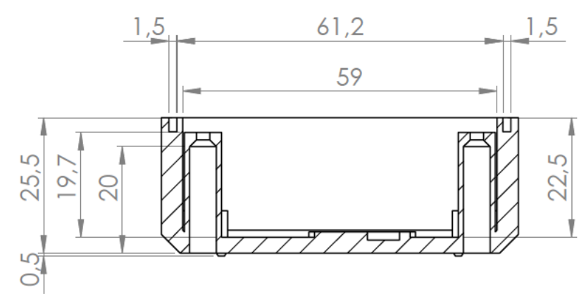
Sección/Section L-L
