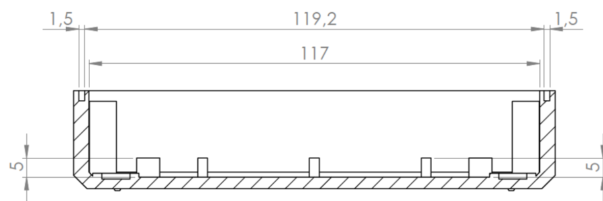
Sección/Section M-M
