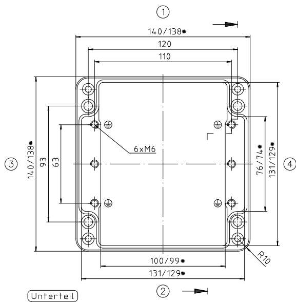
Unterteil
