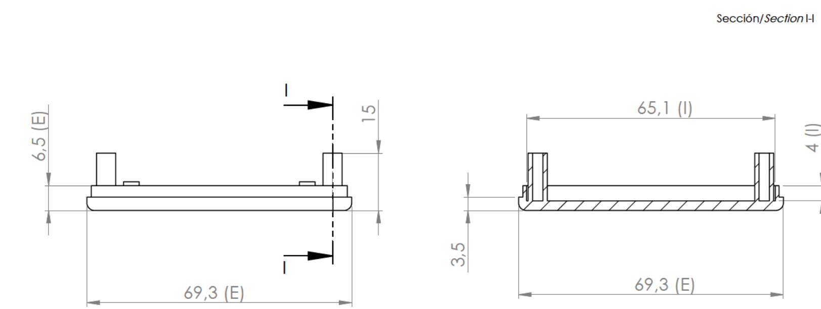
Sección/Section H
