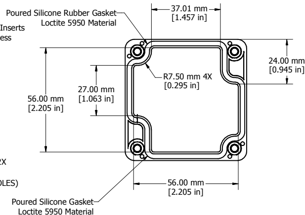
LID - INSIDE
