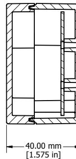
SECTION A-A
