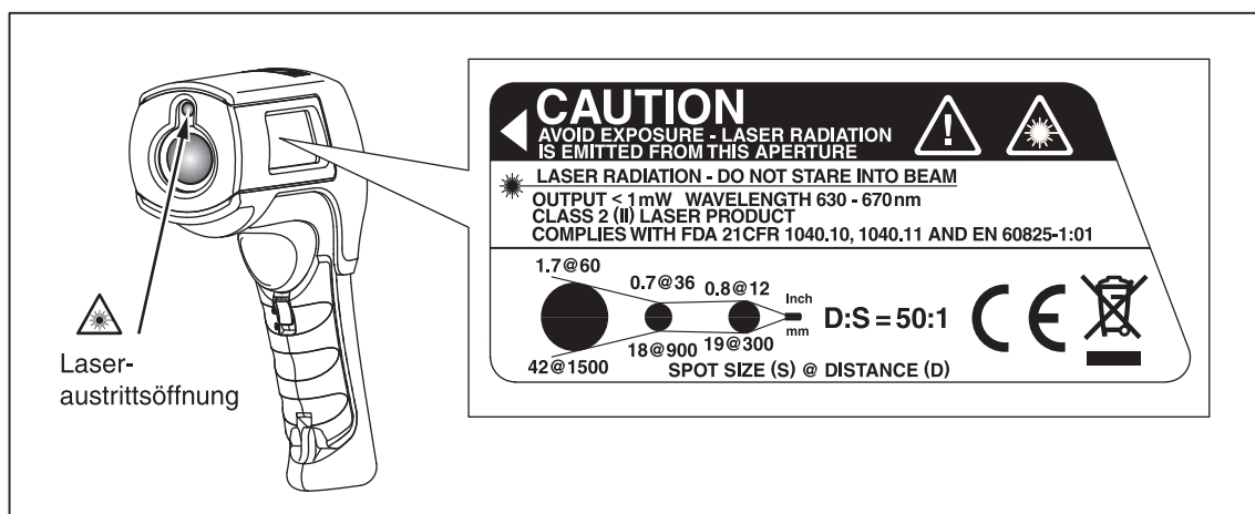
Abbildung 1. Laser-Sicherheitsmarkierungen
