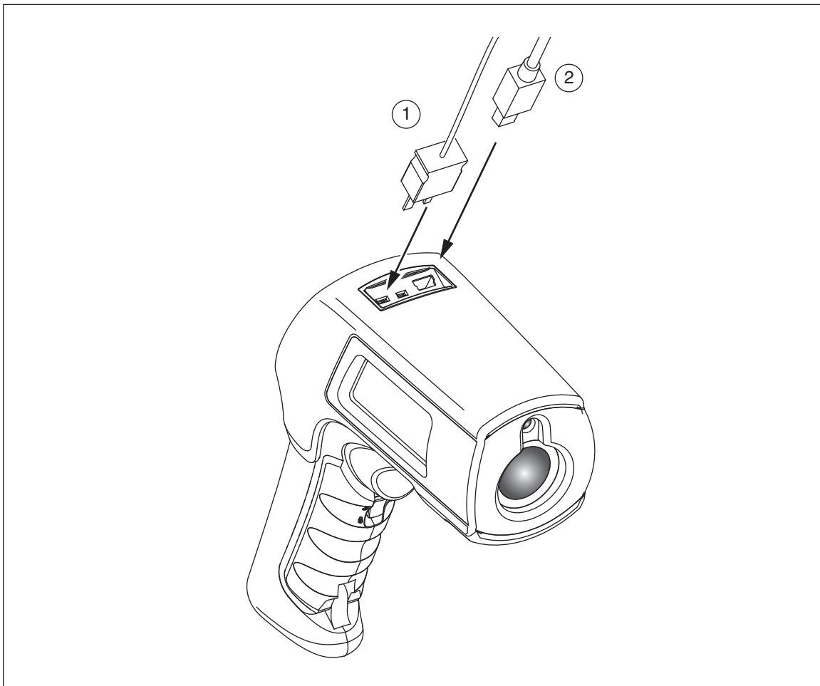
Abbildung 7. Thermoelement- und USB-Anschlüsse
