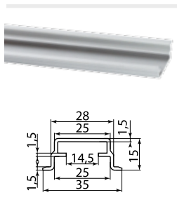
DIN-рейка алюминиевая усиленная 35x15x1,5x2000мм TDM
