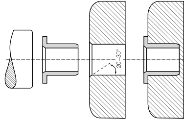
Wykres 21: Wcisk w gniazdo tulei ślizgowych (przekrój poprzeczny)
